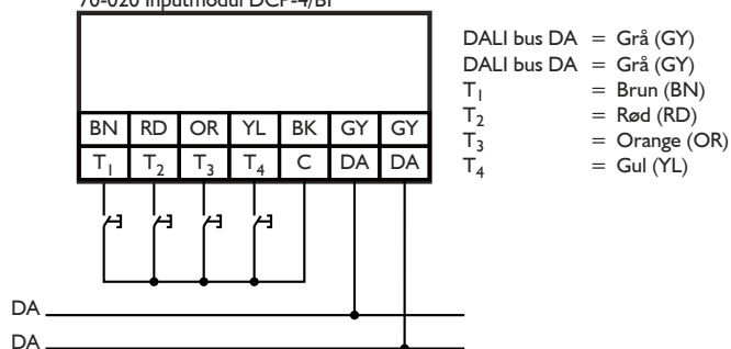
70-020 Inputmodul DCP-4/BI
